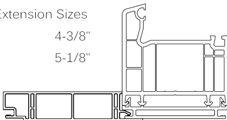
Jamb Extension
